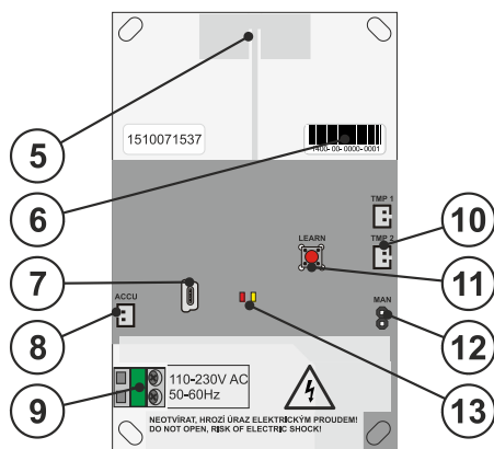
Afbeelding 3: 5 – antenne; 6 – productiecode 7 – mini USB-connector 8 – connector van de back-up batterij; 9 – metaansluitklemmen en beschermfolie;; 10 – connectoren van het sabotagecontact; 11 – knop LEREN; 12 – MAN-klem voor manuele opstart vanuit een back-up batterij; 13 – LED-indicatoren
