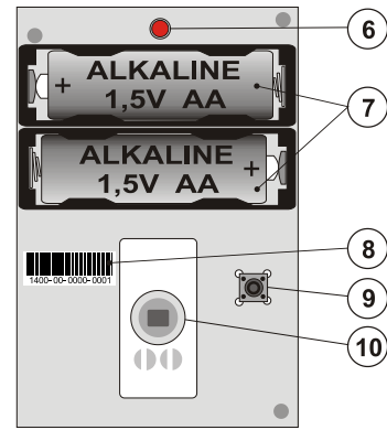
Afbeelding 2: 6 – rode activerings-LED; 7 – batterijen; 8 – Productiecode; 9 – deksel sabotagesensor; 10 – PIR-sensor
