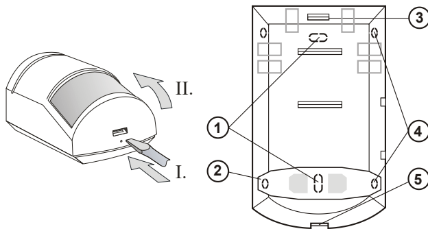
Afbeelding 1: gaten voor installatie op een vlakke muur; 2, 4 – gaten voor installatie onder een hoek (in een hoek); 3 – PCB-tab; 5 – Dekselplijpe
