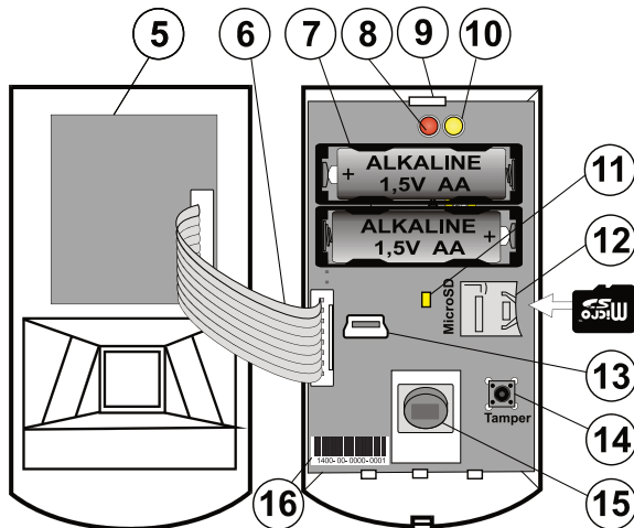
Afbeelding: 5 – Cameramodule; 6 – verbindingkabel; 7 – batterijen; 8 – rode LED indicator; 9 – PCB-tab; 10 – gele LED; 11 – gele LED-indicator van de Micro-SD-kaart; 12 – Micro SD-geheugenkaart; 13 – mini USB-connector; 14 – sabotagecontact; 15 – PIR-sensor; 16 – productiecode.
