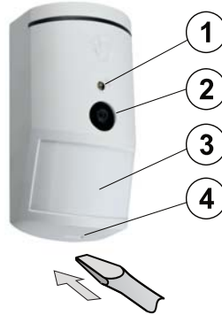
Afbeelding: 1 – flits voor verlichting 2 – cameralens; 3 – lens van de PIR-detector; 4 – deksellijpje;
